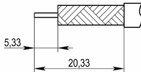
Рисунок 2 Пример разделки кабеля
