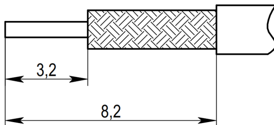
Рисунок 2 Пример разделки кабеля
