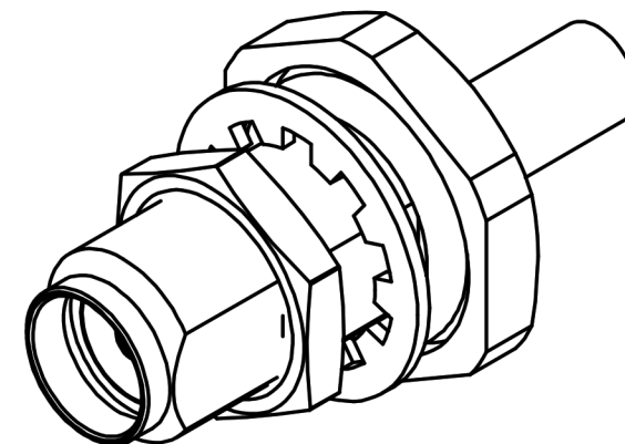
Рисунок 1 АНСШ.434511.139-10 Соединитель СРК-IX-РГ-178-ЦО-1100
