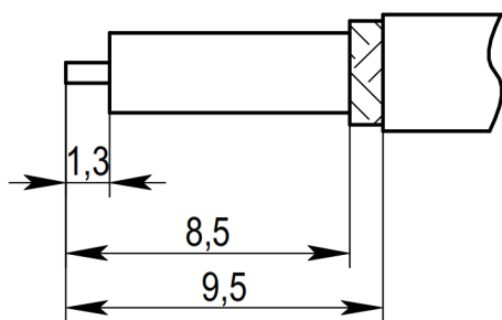
Пример разделки кабеля
